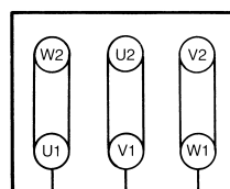
Δ-kobling (lavspenning)
