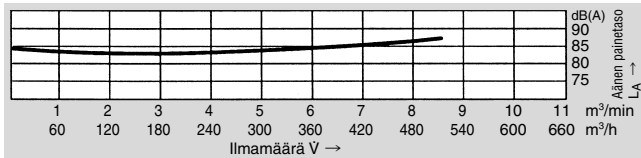
△-kytkentä (matalampi jännite)
