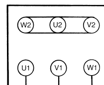
Y-kobling (høyspenning)
