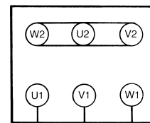
Κύκωμα Υ (μψηλή τάση)
