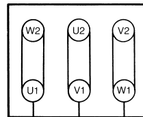
△-kytkentä (matalampi jännite)
