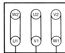
Ligação-Δ (Baixa corrente)
