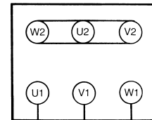
Υ-kytkentä (korkeampi jännite)
