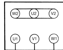
L1 L2 L3 Y-Schaltung (hohe Spannung)
