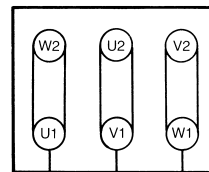
(L3) L2 (L1) △-Schaltung (niedere Spannung)
