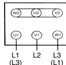
Conexión en estrella (alta tensión)
