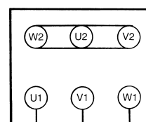
Y-tilslutning (høj spænding)
