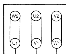
Δ-tilslutning (lav spænding)
