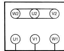
Conexión en estrella (alta tensión)
