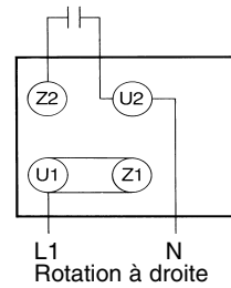
Rotation à droite
