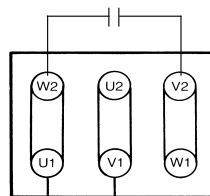
L1 N Obroty w prawo
