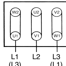
Conexión de triángulo (baja tensión)
