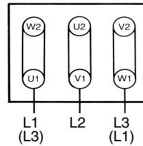
Couplage \Delta (tension basse)
