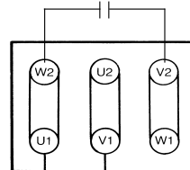
Rotación a derechas
