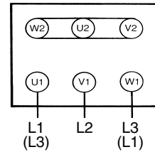
Couplage Y (tension haute)
