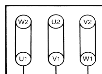
L1 L2 L3 (L3) (L1) Połączenie w trójkąt (niskie napięcie)
