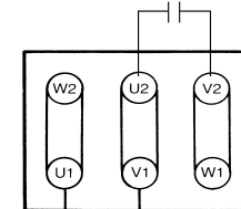
Rotación a izquierdas
