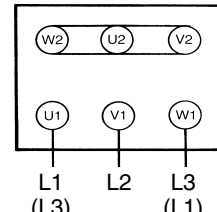
Conexión en estrella (alta tensión)
