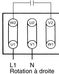
Rotation à droite
