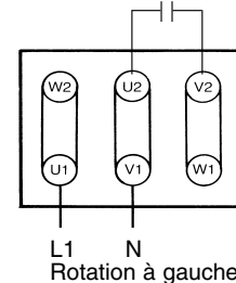
Rotation à gauche
