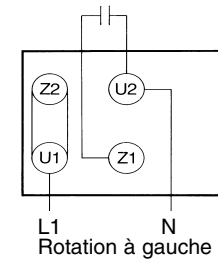
Rotation à gauche
